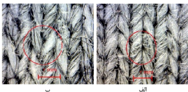
شکل ۶ نمایشی از شکل حلقه با بزرگنمایی ۵۰ برابر، (الف) نمونه خشک (ب) نمونه خیس
