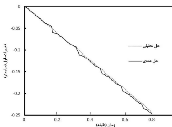
شکل ۵ مقایسه بین حل عددی و حل تحلیلی
