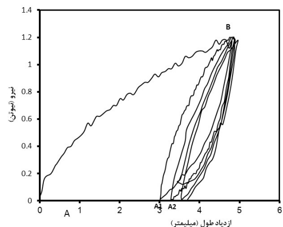
شکل ۹ نمودار هیستریزس نمونه ۱
